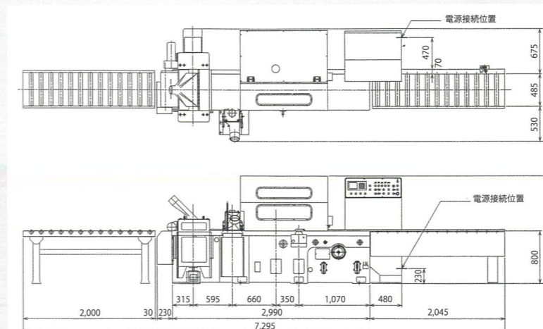
図面: KFP-S500型
